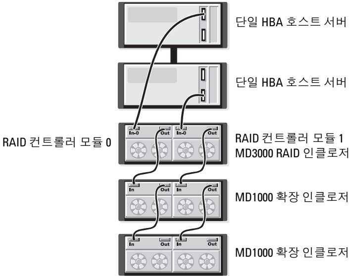
그림 2-3. 2 노드 클러스터(단일 HBA, 각 노드에서 비중복 데이터 경로) 케이블링
