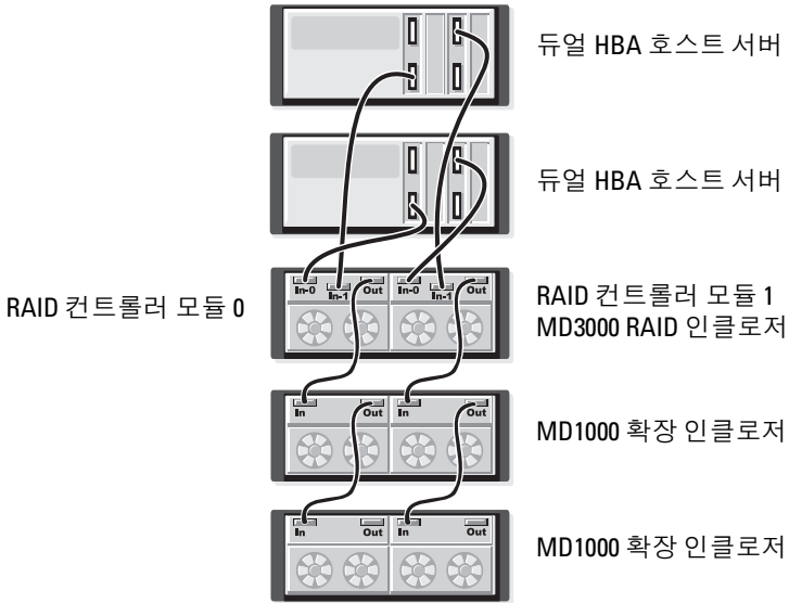
그림 2-9. 중복 데이터 경로를 사용하여 두 호스트(듀얼 HBA) 케이블링
