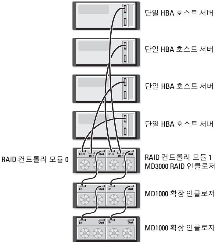
그림 2-6. 비중복 데이터 경로로 최대 네 개의 호스트 케이블링
