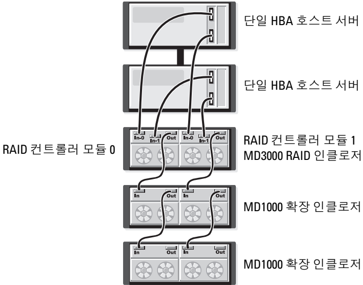
그림 2-11. 2 노드 클러스터(단일 HBA, 각 노드의 중복 데이터 경로) 케이블링
