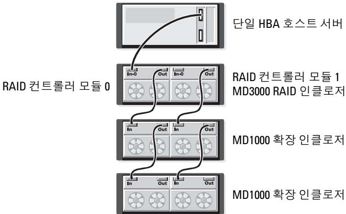
그림 2-1. 비중복 데이터 경로로 하나의 호스트 케이블링
