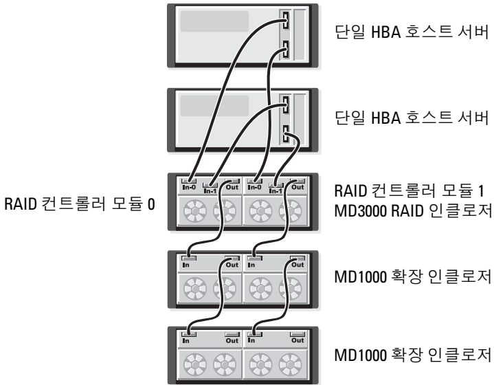
그림 2-10. 중복 데이터 경로를 사용하여 두 호스트(단일 HBA) 케이블링
