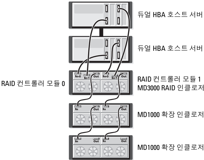
그림 2-12. 2노드 클러스터(단일 HBA, 각 노드의 중복 데이터 경로) 케이블링
