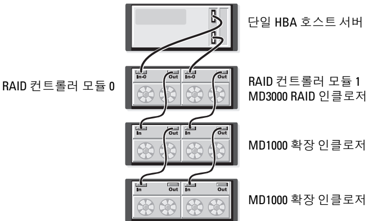
그림 2-5. 중복성 데이터 경로를 사용하여 단일 호스트(단일 HBA) 케이블링
