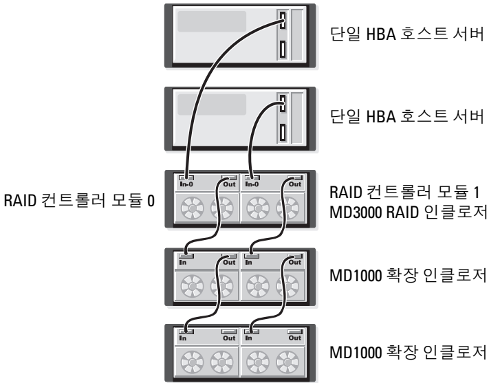
그림 2-2. 비중복 데이터 경로로 두 개의 호스트 케이블링
